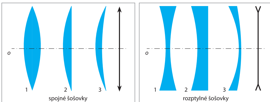
Obr. 35 Druhy šošoviek a ich značky
