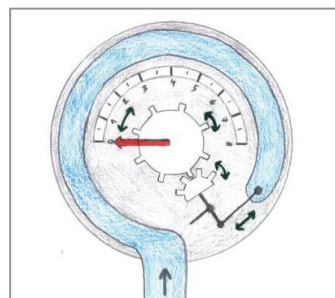
Obr. 96 Deformačný manometer
