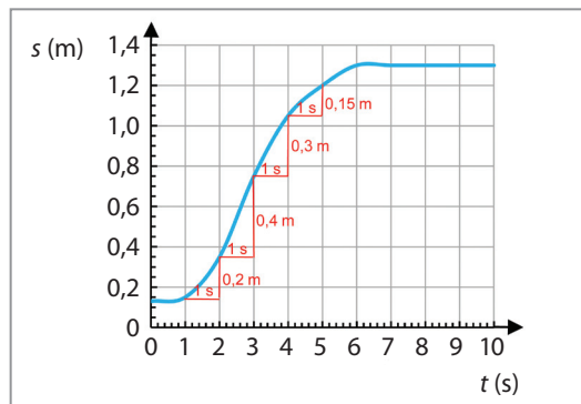
Obr. 108 Graf závislosti dráhy od času
