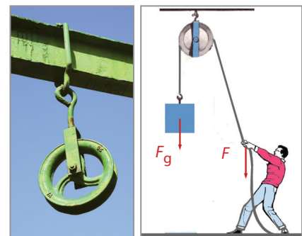
Obr. 120 Pevná kladka
