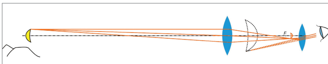
Obr. 56 Schéma pozorovania Mesiaca ďalekohľadom
