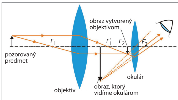
Obr. 55 Zobrazenie ďalekohľadom
