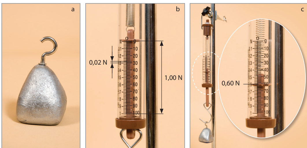
Obr. 69 a) Teleso, ktoré meriame. b) Jeden dielik zobrazuje veľkosť 0,02 N, rozsah silomeru je 1,00 N. c) Odmeraná hodnota F = 0,60 \text{ N} \pm 0,02 \text{ N}
