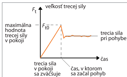
Obr. 99 Graf závislosti veľkosti trecej sily od času pri pohybe kvádra po podložke
