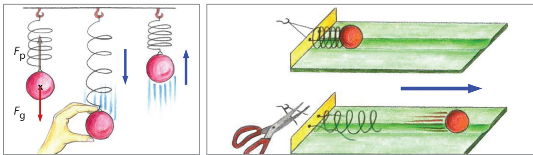
Obr. 127 Polohová energia pružnosti pružiny
