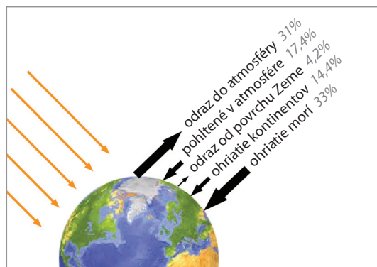
Obr. 131 Diagram energie vysielanej zo Slnka na Zem
