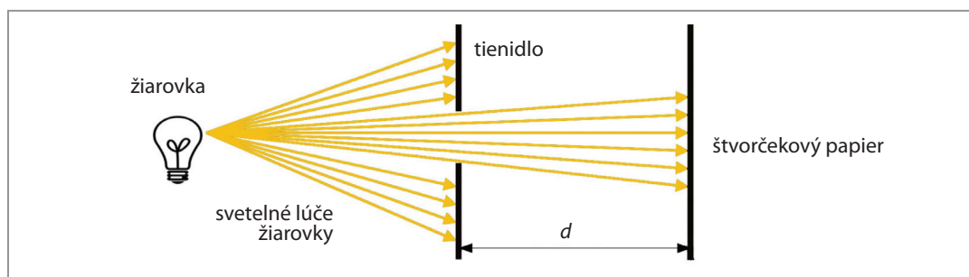
Obr. 10 Plocha osvetlená rozbiehavými lúčmi zo žiarovky
