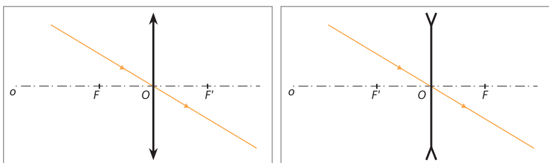
Obr. 40 Lúč prechádzajúci optickým stredom šošoviek
