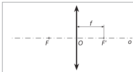
Obr. 37 Dôležité charakteristiky spojky
