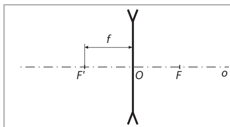
Obr. 39 Dôležité charakteristiky rozptylky
