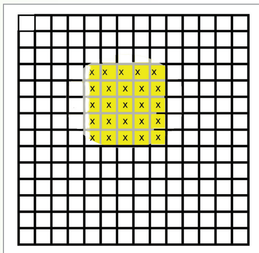
Obr. 8 Meranie plochy osvetlenej svetlom žiarovky
