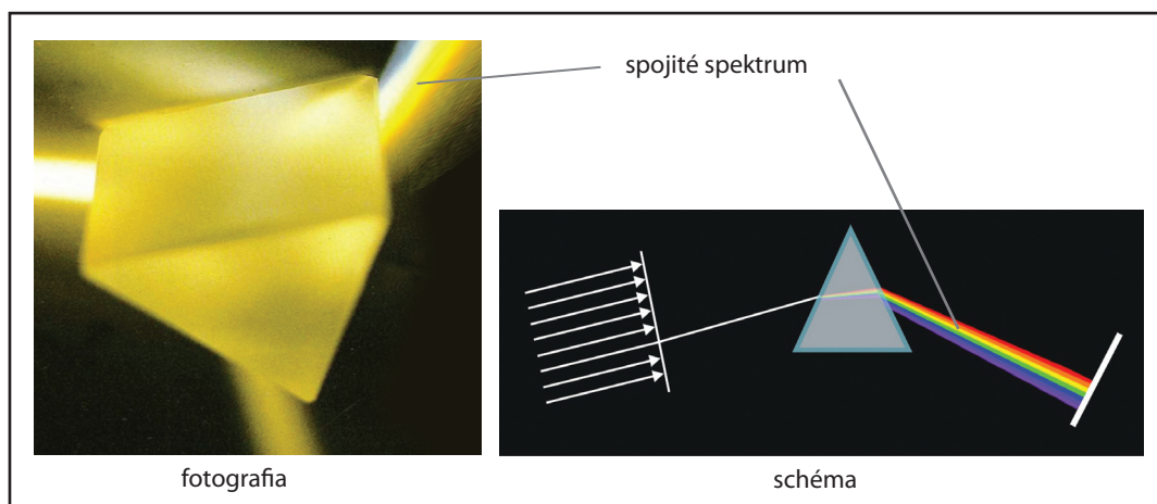
Obr. 14 Rozklad svetla hranolom
