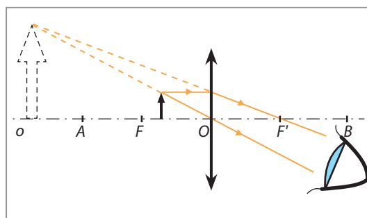
Obr. 47 Zobrazenie predmetu spojnou šošovkou vo vzdialenosti menšej ako f
