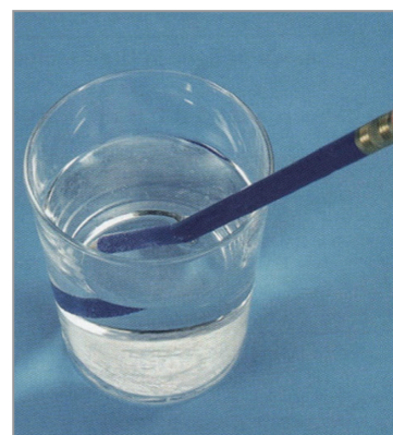
Obr. 28 Pohľad na ceruzku ponorenú vo vode
