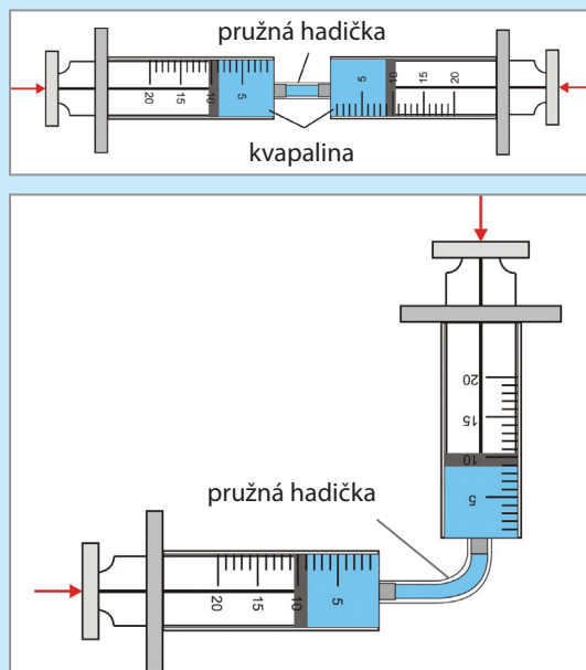
Obr. 84 Kvapaliny sú nestlačiteľné. Tlak spôsobený vonkajšou silou sa prejavuje v celom objeme kvapaliny
