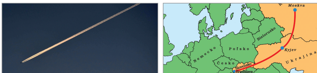
Obr. 105 Trajektória letu lietadla vo vzduchu a na mape
