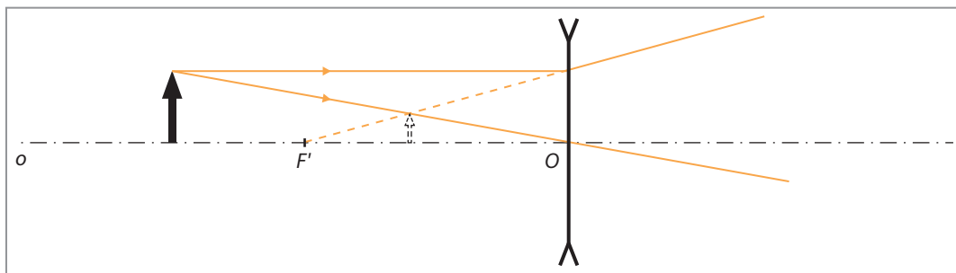
Obr. 48 Zobrazenie predmetu rozptylnou šošovkou
