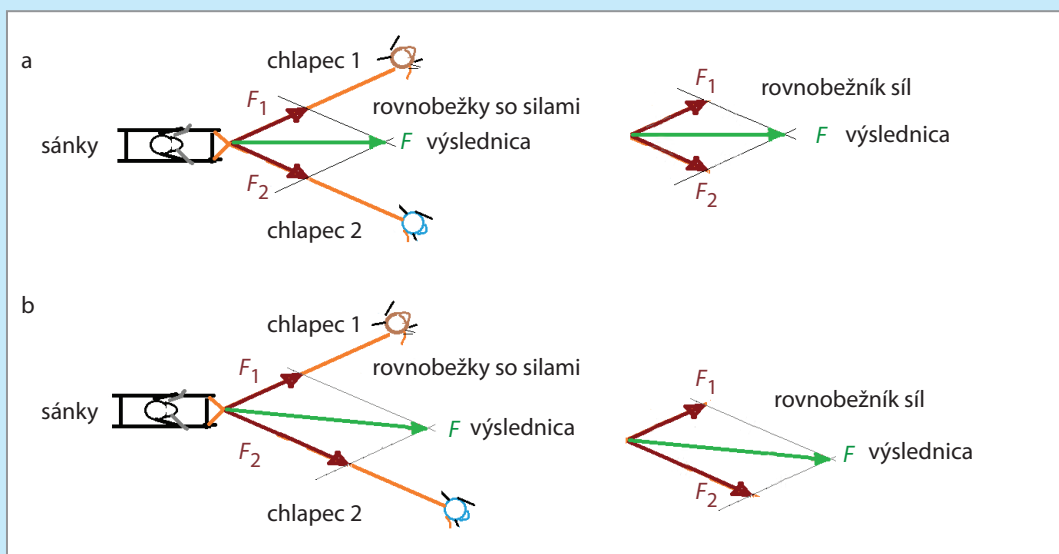
Obr. 75 Skladanie síl pomocou rovnobežníka
