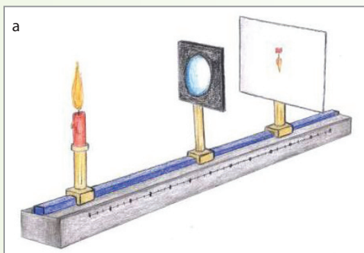
Obr. 44 Zobrazenie plameňa sviečky v rôznej vzdialenosti od lupy
