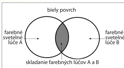
Obr. 17 Skladanie farebných svetelných lúčov
