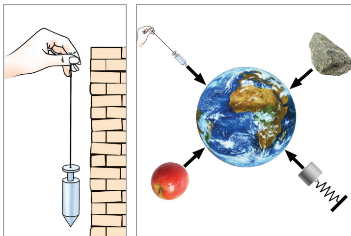
Obr. 65 Určovanie zvislého smeru
