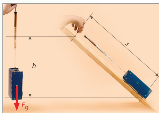
Obr. 119 Konanie práce ťahaním vozíka po naklonenej rovine a jeho dvíhaním zvisle nahor
