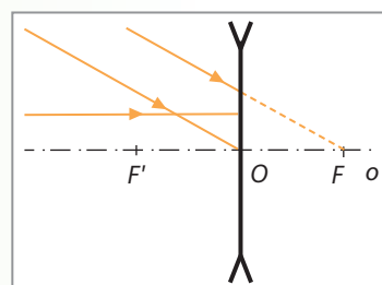
rozptylka
