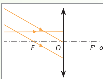
spojka
