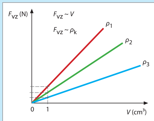
Obr. 86 Graf závislosti medzi veľkosťou vztlakovej sily a objemom telesa ponoreného v kvapalinách s rôznou hustotou \rho
