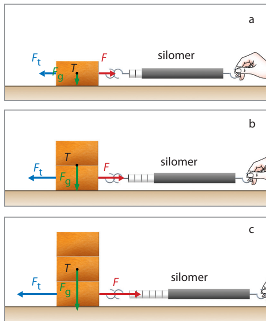
Obr. 101 Meranie trecej sily v závislosti od tlakovej sily, ktorou teleso pôsobí na podložku (jeden, dva alebo tri kvádre)
