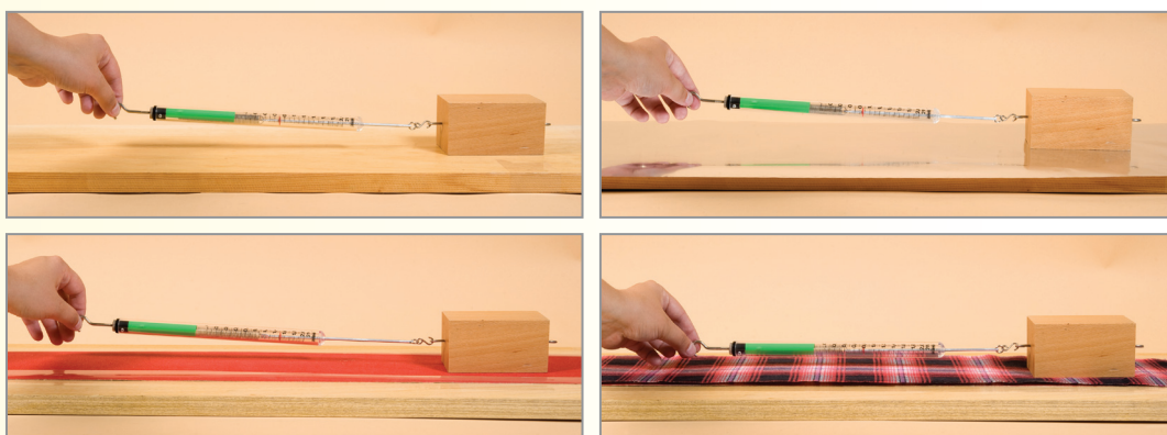
Obr. 97 Meranie trecej sily tesne pred pohybom a v priebehu pohybu kvádra po podložkách
