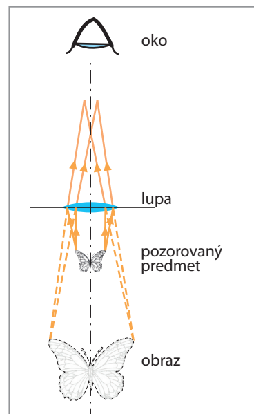
Obr. 53 Zväčšenie lupou
