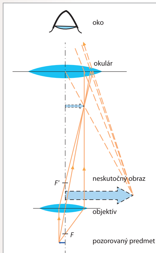
mikroskop
