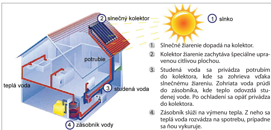
Obr. 135 Schéma kolektora na ohrev vody
