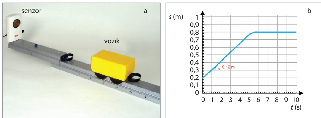
Obr. 107 Záznam pohybu vozíka pomocou senzora a grafického zobrazenia na počítači
