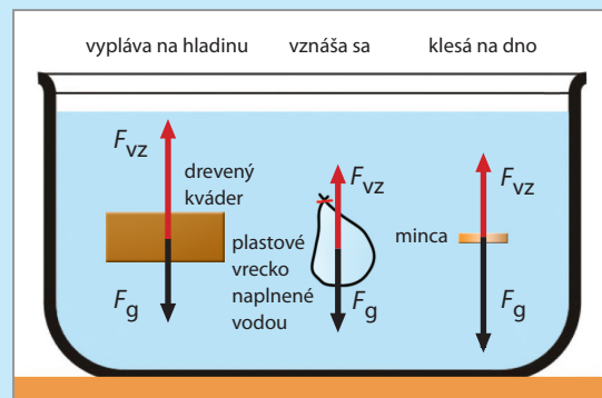
Obr. 88 Poloha telies v kvapaline na začiatku myšlienkového experimentu
