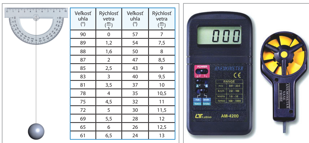
Obr. 111 Žiacký anemometer a tabuľka na zisťovanie rýchlostí, digitálny anemometer
