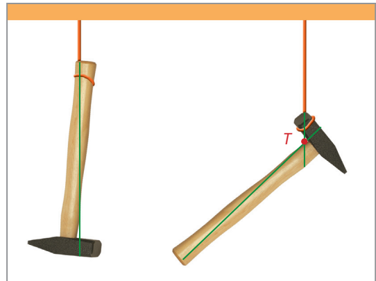
Obr. 79 Posunutie ťažiska smerom k časti s väčšou hustotou
