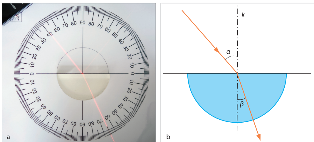
Obr. 29 Prechod svetelného lúča zo vzduchu do skla
