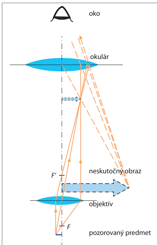
Obr. 58 Zobrazenie mikroskopom
