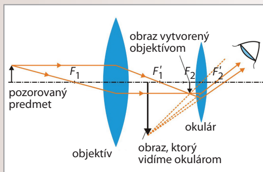
ďalekohľad
