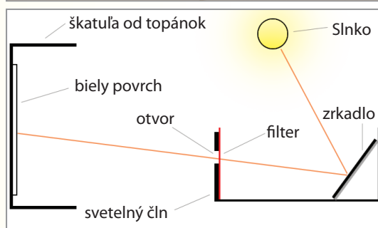
Obr. 16 Schéma zariadenia na skladanie farebných svetelných lúčov
