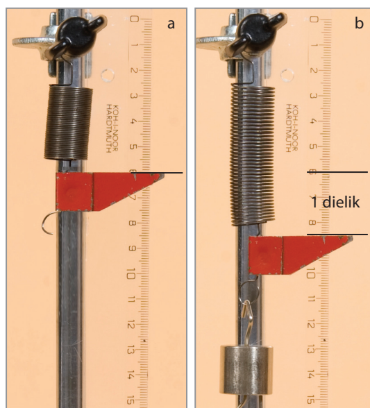
Obr. 67 Pružinový silomer a základ merania pružinovým silomerom
