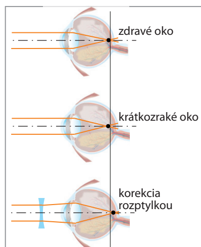
Obr. 50 Krátkozraké oko a odstránenie jeho chyby
