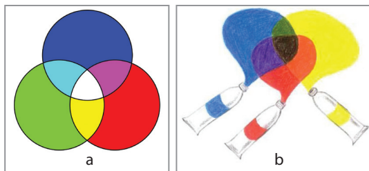
Obr. 18 Skladanie farebných svetelných lúčov a miešanie náterových farieb
