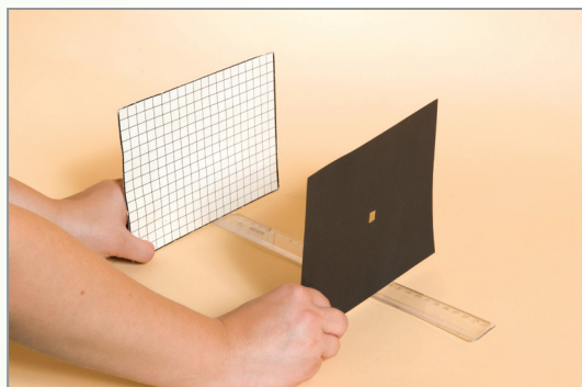
Obr. 7 Meranie plochy osvetlenej slnečným svetlom
