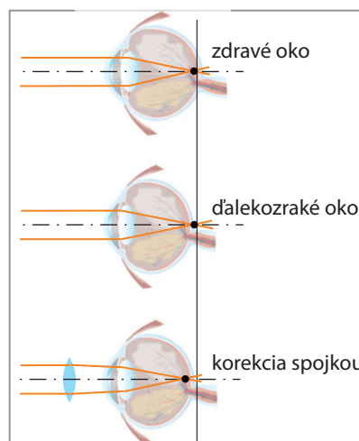
Obr. 51 Ďalekozraké oko a odstránenie jeho chyby
