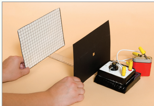
Obr. 8 Meranie plochy osvetlenej svetlom žiarovky
