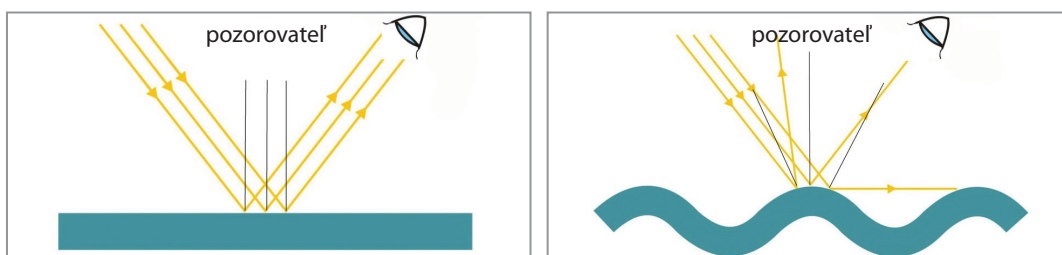
Obr. 25 Odraz svetla od vodorovnej lesklej plochy a od nerovnej plochy
