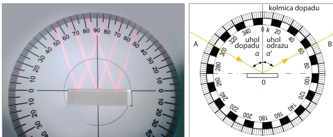
Obr. 24 Zobrazenie odrazu svetla a schematické znázornenie lúčov
