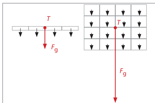
Obr. 77 Výslednica síl, ktorými Zem pôsobí na jednotlivé časti telesa
