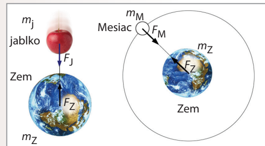
Prostredníctvom gravitačného poľa
