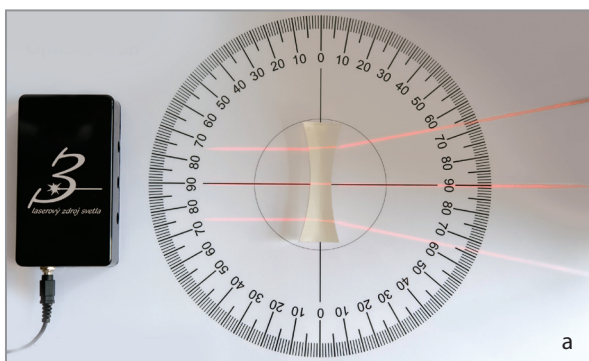
Obr. 38 a) Modelový experiment s rozptylkou na optickom kruhu
