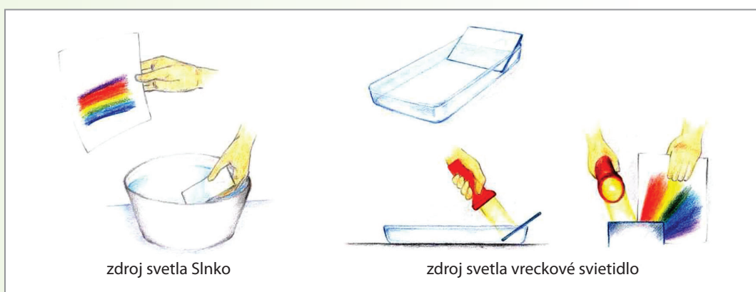
Obr. 13 Schéma pokusu s rozkladom svetla
