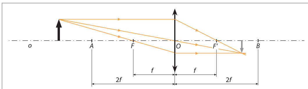
Obr. 45 Zobrazenie predmetu spojnou šošovkou vo vzdialenosti väčšej ako 2f
