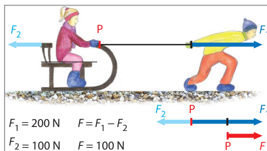
Obr. 72 Skladanie síl v opačnom smere
