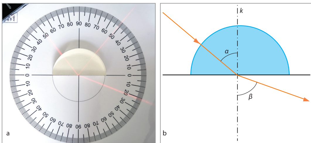
Obr. 30 Prechod svetelného lúča zo skla do vzduchu
