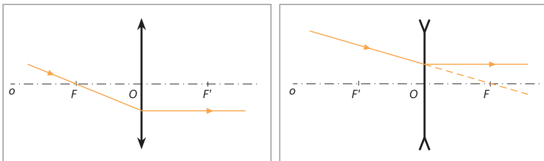
Obr. 41 Lom lúča, ktorý prechádza ohniskom spojenej šošovky a lom lúča, ktorý smeruje do ohniska rozptylnej šošovky
