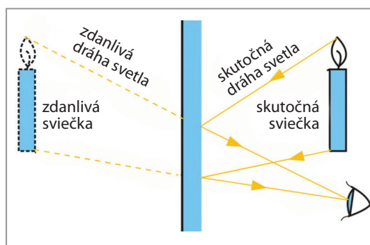
Obr. 26 Zostrojenie obrazu v zrkadle
