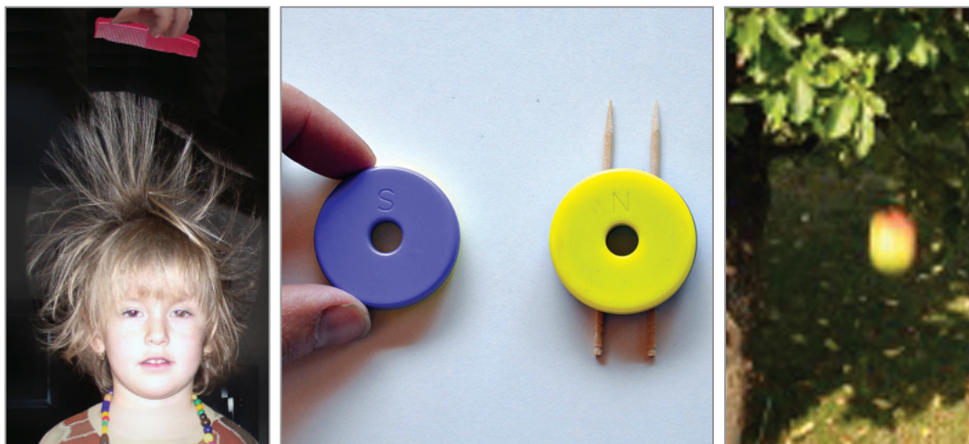
Obr. 61 Pôsobenie sily medzi telesami bez priameho kontaktu
