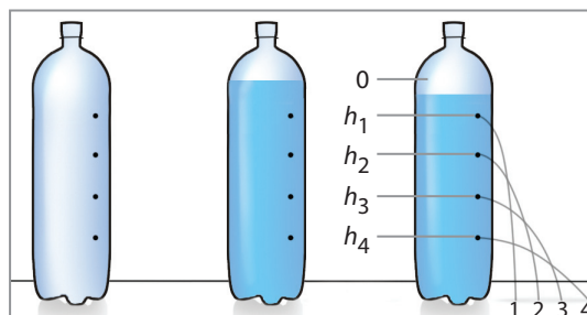
Obr. 91 Overenie súvislosti medzi hydrostatickým tlakom a hĺbkou h kvapaliny
