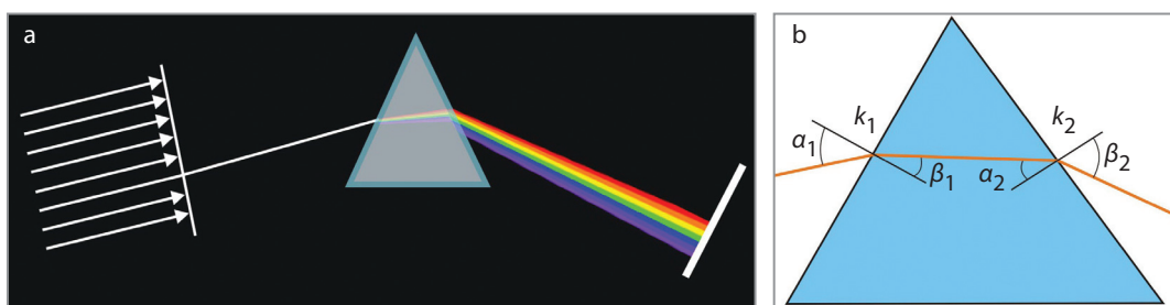
Obr. 33 Schéma rozkladu svetla hranolom
