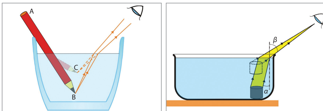
Obr. 31 Vysvetlenie pozorovania ceruzky ponorenej v pohári s vodou
