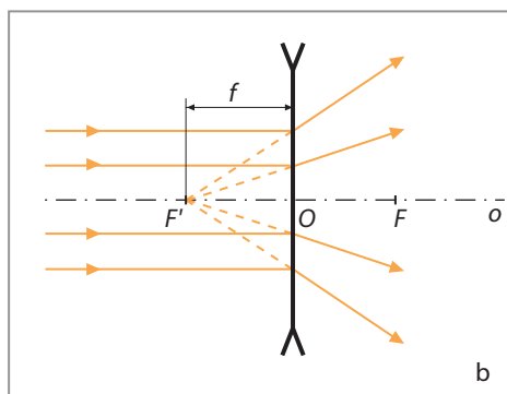
b) Rovnobežné svetelné lúče prechádzajúce rozptylkou
