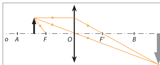
Obráz je skutočný, prevrátený a zväčšený
