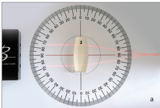
Obr. 36 a) Modelový experiment so spojkou na optickom kruhu
