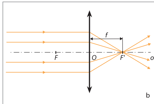
b) Rovnobežné svetelné lúče prechádzajúce spojkou
