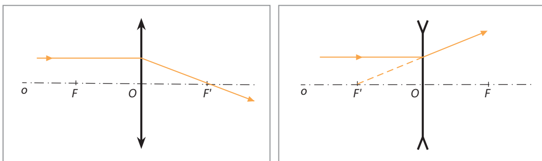
Obr. 42 Lom lúča rovnobežného s optickou osou
