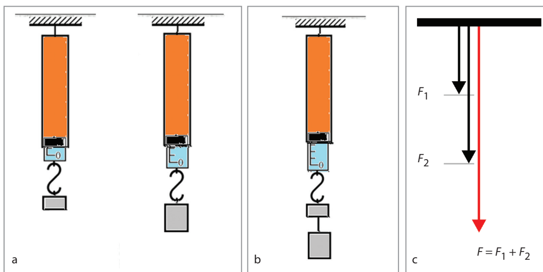
Obr. 71 Skladanie dvoch síl rovnakého smeru
