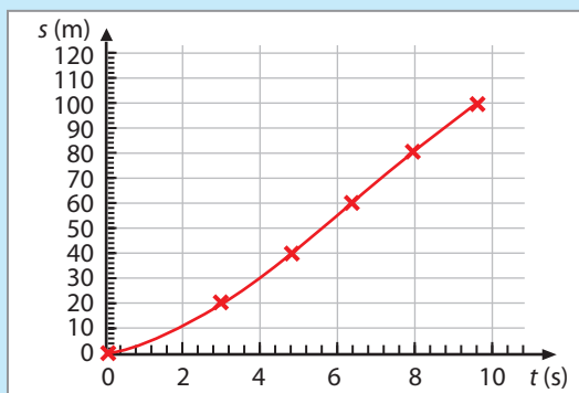
Graf A – závislosť dráhy od času pri behu športovca na 100 m
