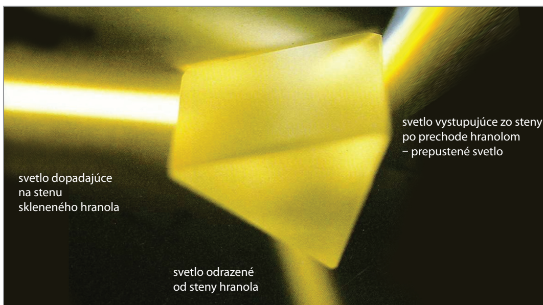
Obr. 11 Správanie svetla dopadajúceho na sklenený hranol
