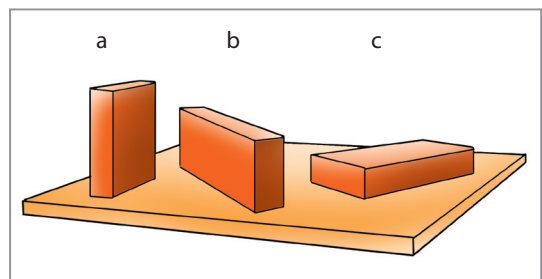
Obr. 81 Stálosť polohy - stabilita
