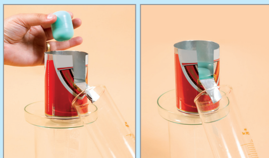
Obr. 87 Objem vody vytlačenej telesom
