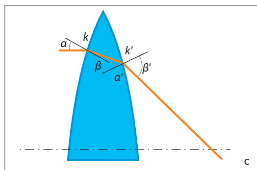
c) Lom svetelného lúča prechádzajúceho spojkou
