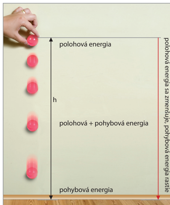
Obr. 130 Premena energie pri páde loptičky
