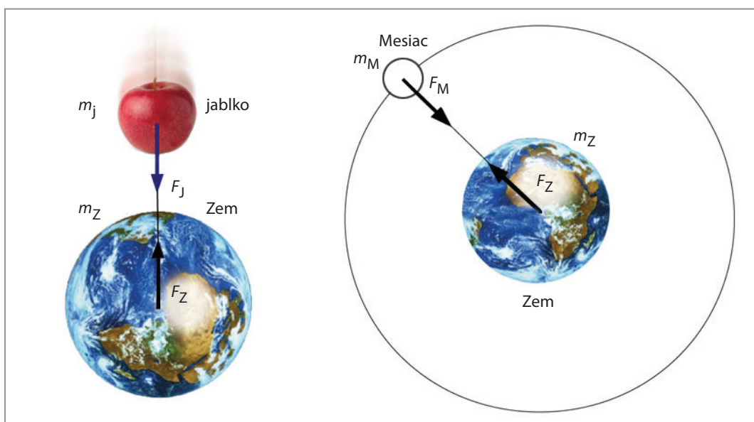
Obr. 62 Silové pôsobenie medzi telesami je vzájomné
