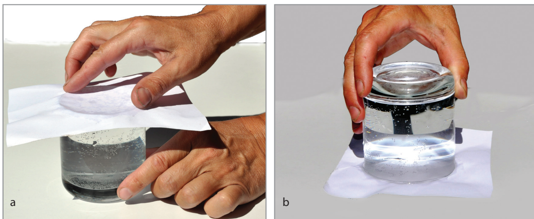
Obr. 93 Dôkaz pôsobenia tlakovej sily v atmosfére
