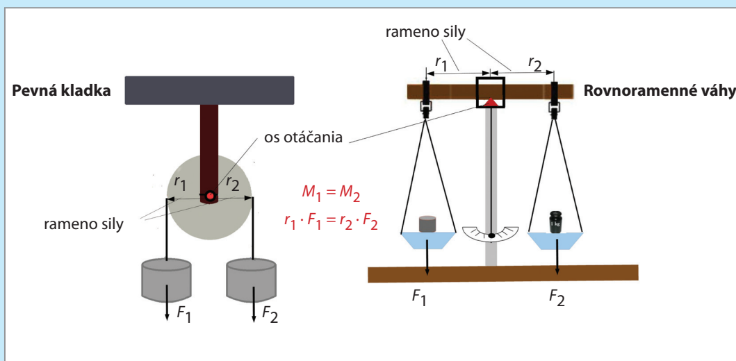
Obr. 123 Porovnanie pevnej kladky a rovnoramennej páky, v našom prípade rovnoramenných váh
